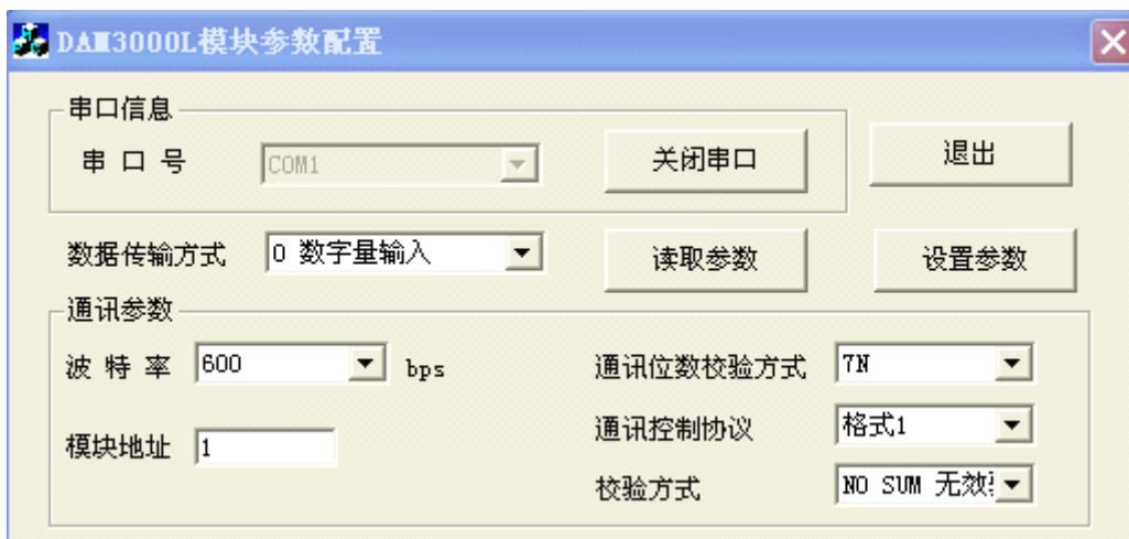
（图 10）DAM-3000L 模块参数配置界面
