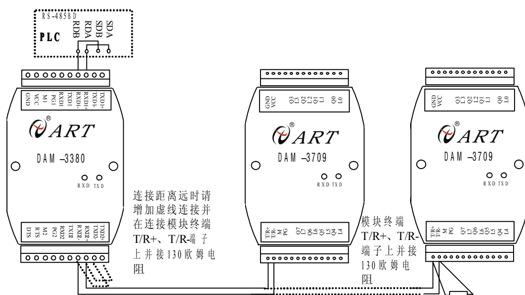
（图 6）DAM-3709 连接图
