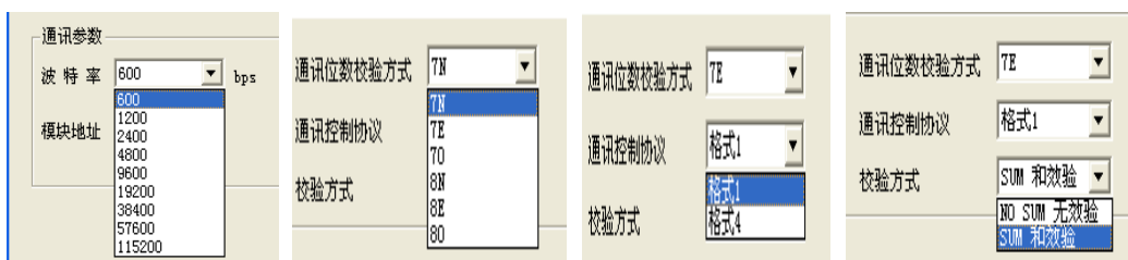
(图 12) DAM-3000L 模块参数配置界面
