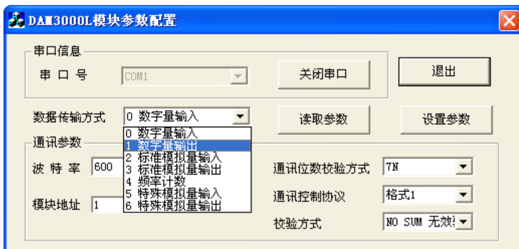
(图 11) DAM-3000L 模块参数配置界面
