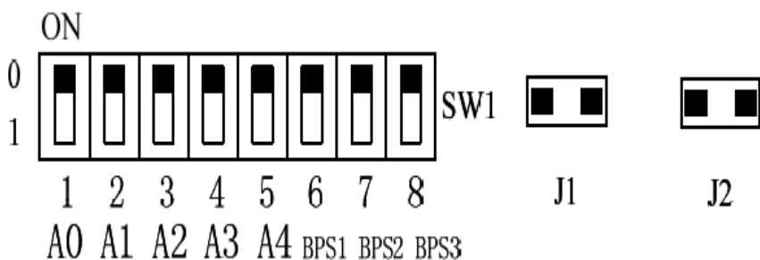
(图 8) 手动配置参数示意图
