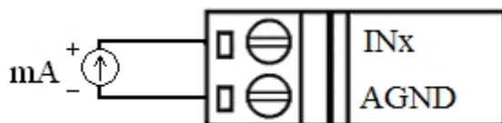
模拟量输入接线图
