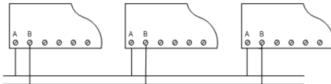
(图 1) 单总线连接
