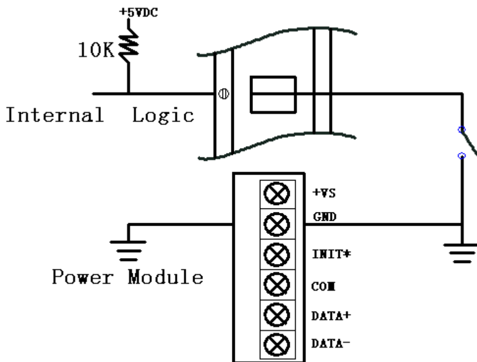
湿接点接线（外接 0~30V 电压）
