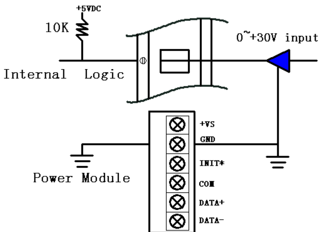
湿接点接线（外接 0~30V 电压）
