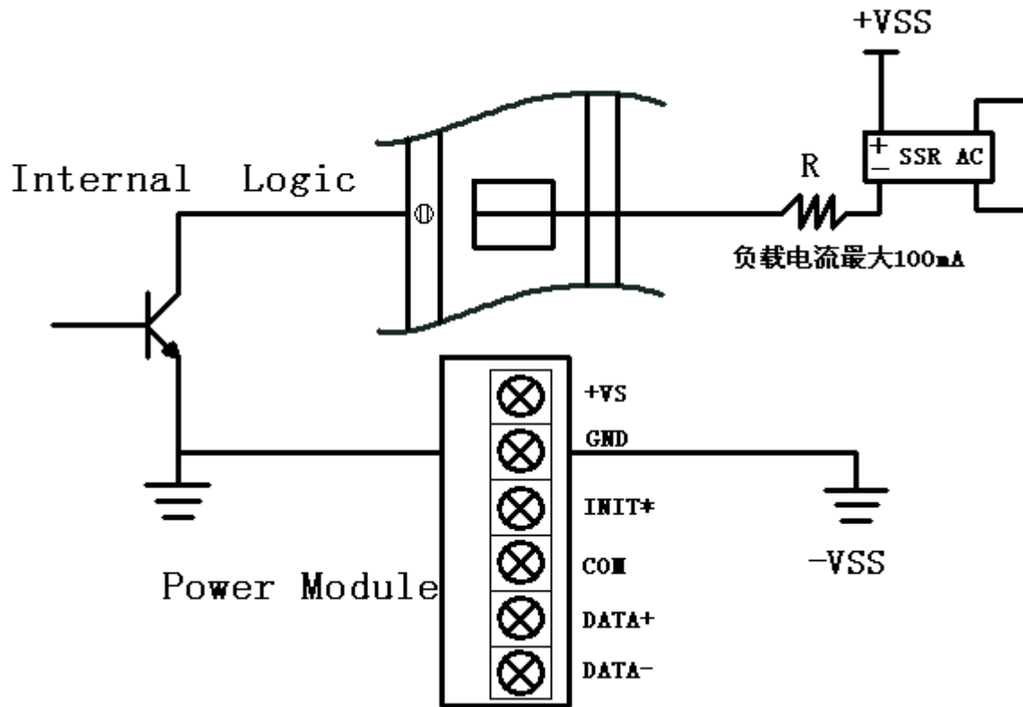
外接电路图（DO 通过电阻 R 接到 0~30V 电源正端，电源负端接到电源板的 GND 脚）
