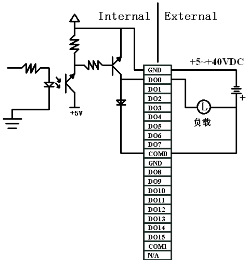
外部接线图（负载电流最大 200mA）
