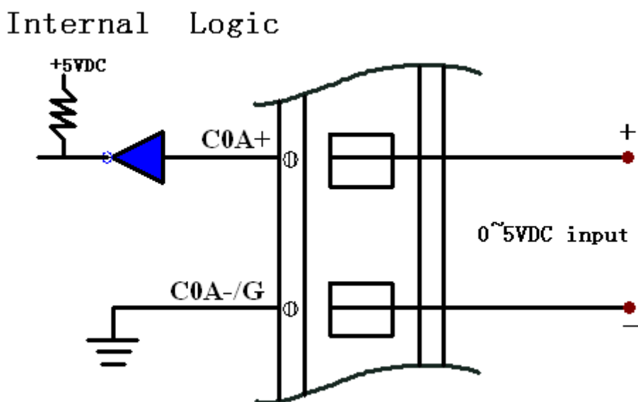
非隔离状态接线（B 信号同 A 信号）
