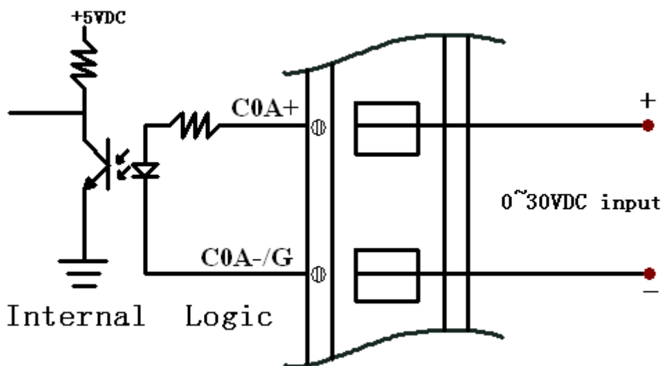
隔离状态接线（B 信号同 A 信号）
