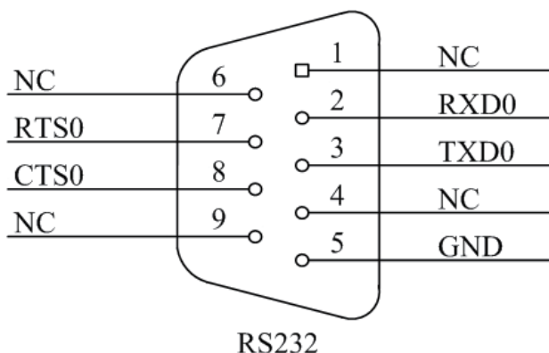
RS232/RS485/DEBUG串口COM2定义
