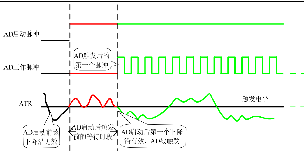
5.3 下降沿触发图例
