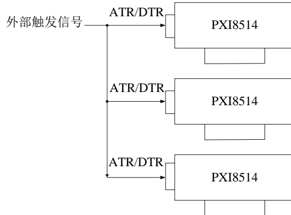
外触发同步采集的连接方法
