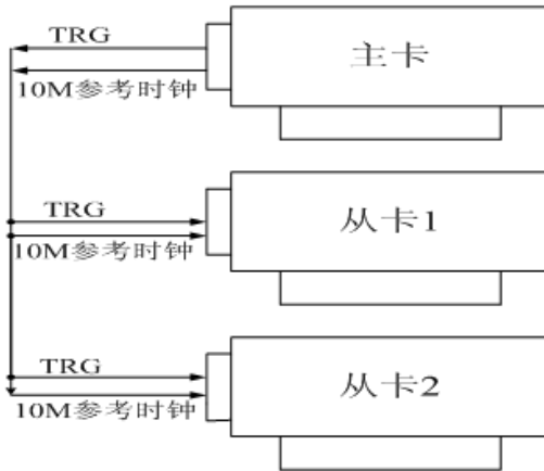
多卡级联的连接方法
