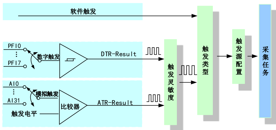
图 8-1-1 触发源选择
