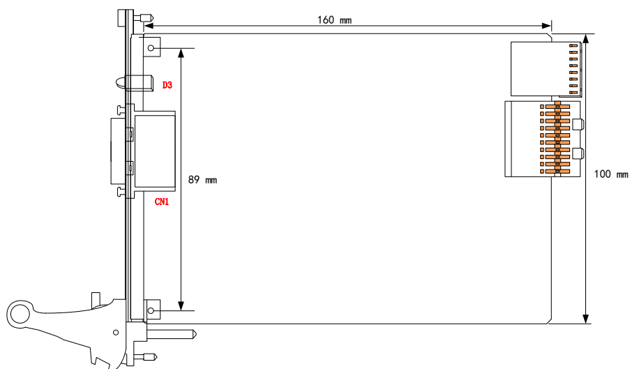
图 3-2-1 外壳尺寸图
