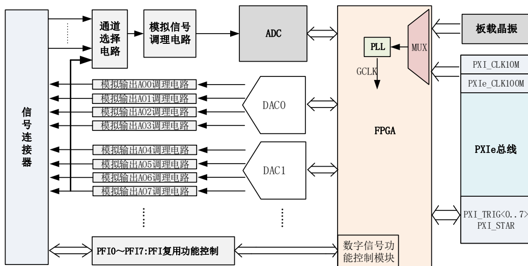
图2-2-1 PXIe9320系统框图
