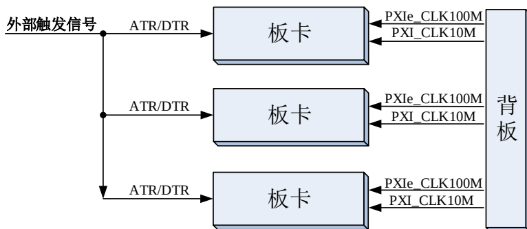
图 4-10-1 主从卡级联
