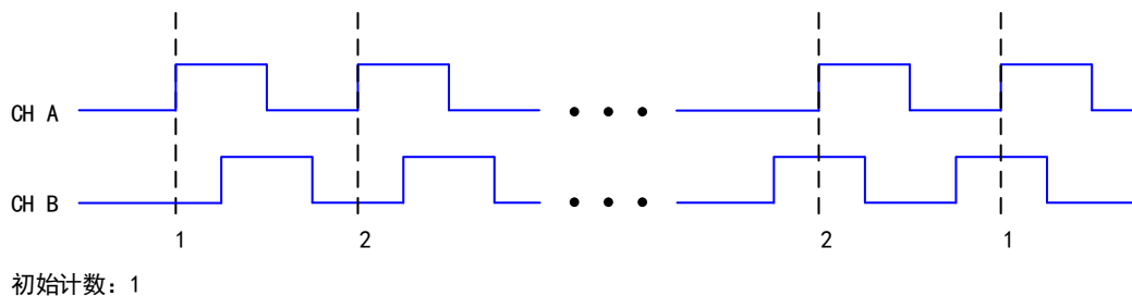
图 6-6-1 X1 编码
