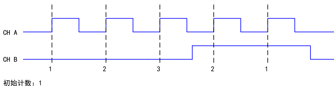
图 6-6-5 单脉冲编码
