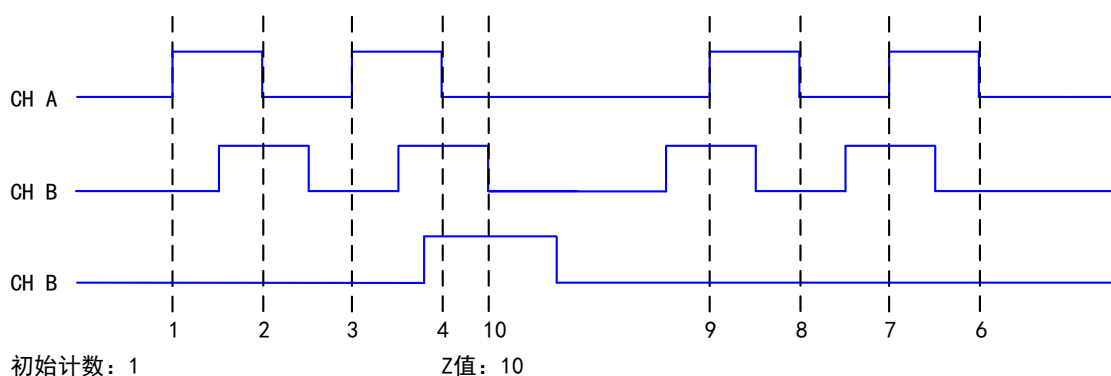
图 6-6-6 Z 索引
