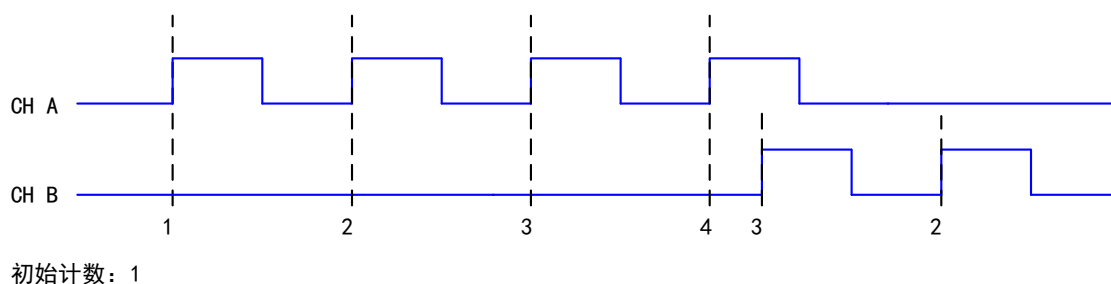
图 6-6-4 双脉冲编码
