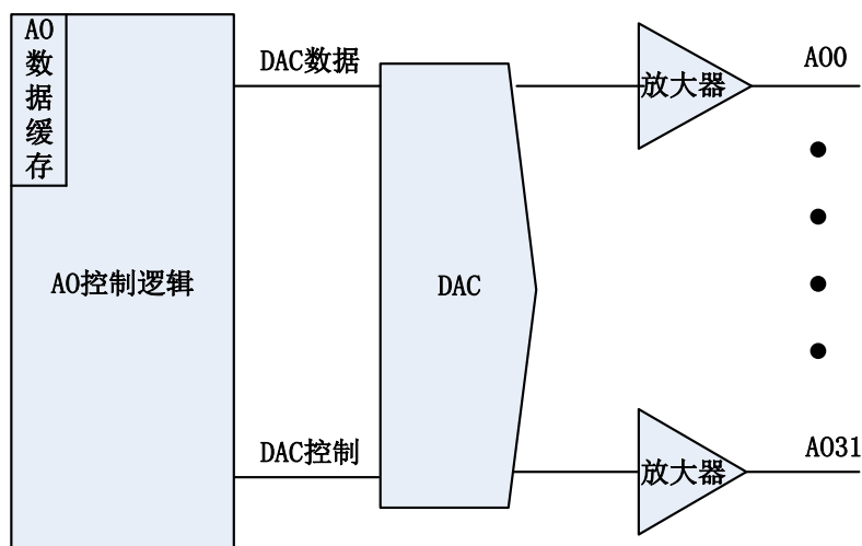
图 5-1-1 AO 功能框图
