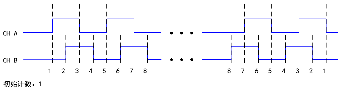
图 6-6-3 X4 编码
