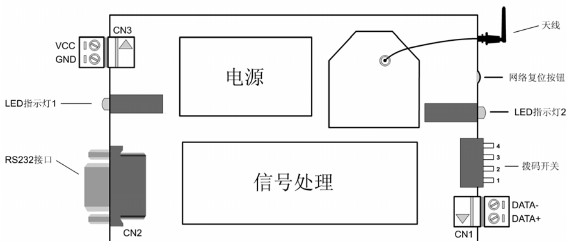
ZIGBEE1080A模块结构及接线端子图
